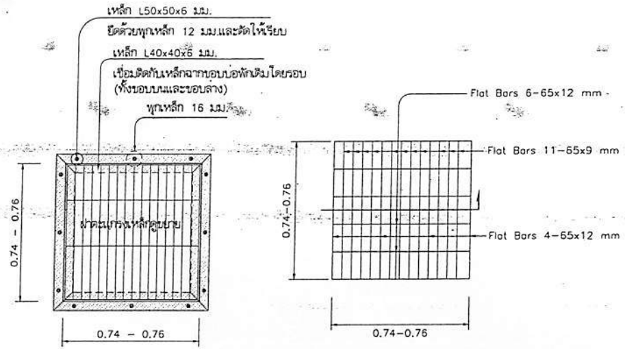
แบบส่นบ่อพัก A 1:20
