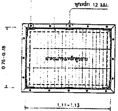
แปลนบ่อพัก 1:20
