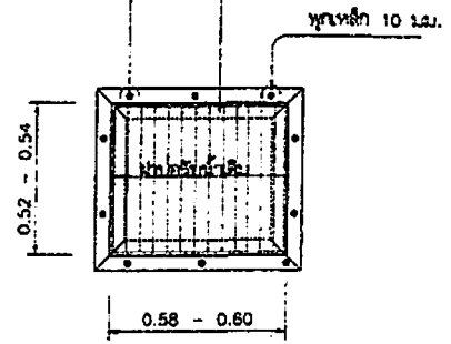
แปลนบ่อรับน้ำ 1:20
