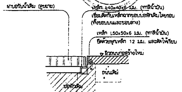
รูปตัด 1:10
