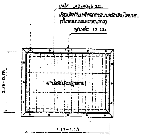
แปลนบ่อพัก 1:20
