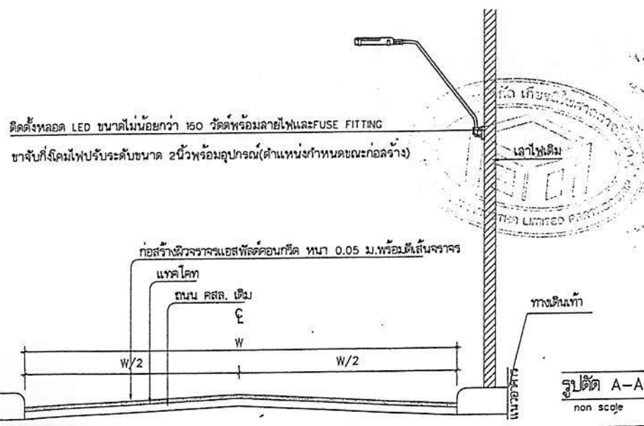
ขยายงานดีเส้นจรวจร ไม่แสดงขนาดส่วน
