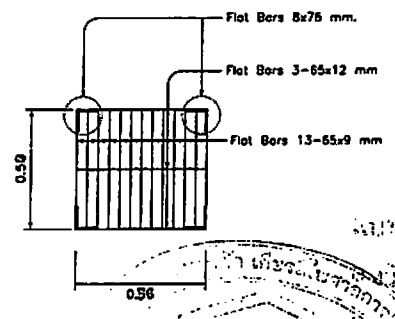
ขยายผ่านบ่อรับน้ำ 1:25
