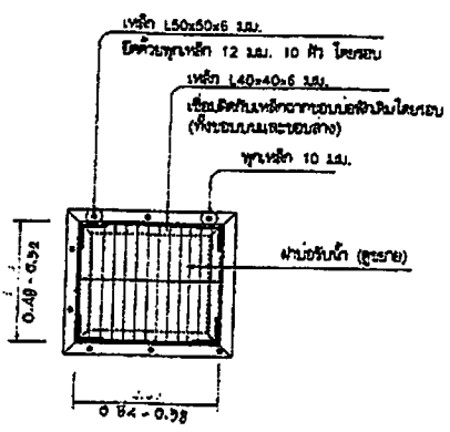
แปลนบ่อรับน้ำ 1:25
