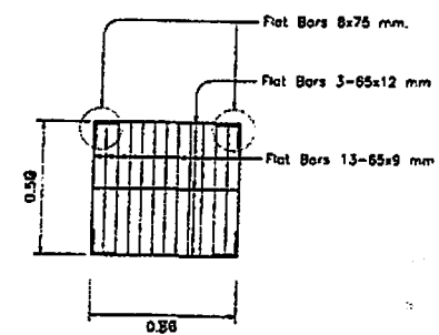
ขยายฝาบ่อรับน้ำ 1:25
