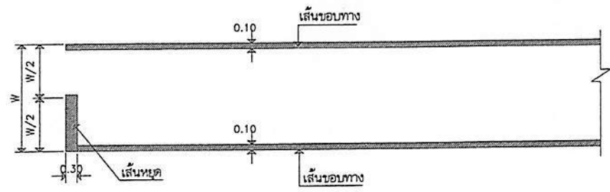
ขยายงานดีเส้นจรวจร ไม่แสดงขนาดส่วน
