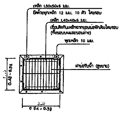
แปลนบ่อรับน้ำ 1:25
