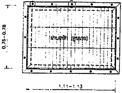
แปลนบ่อพัก 1:20
