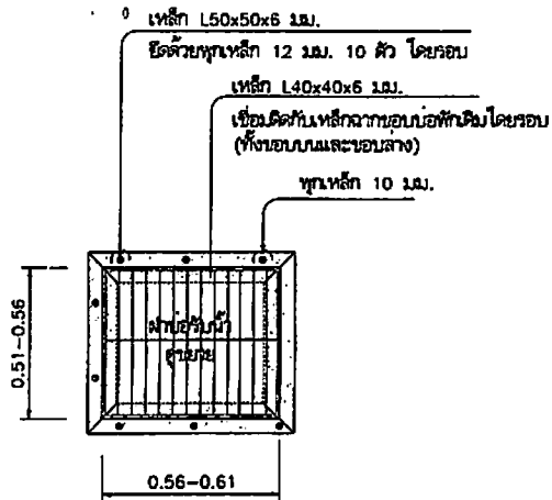
แบบบ่อรับน้ำ 1:20
