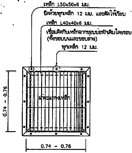
แบบสกรีนบ่อพัก 1:20
