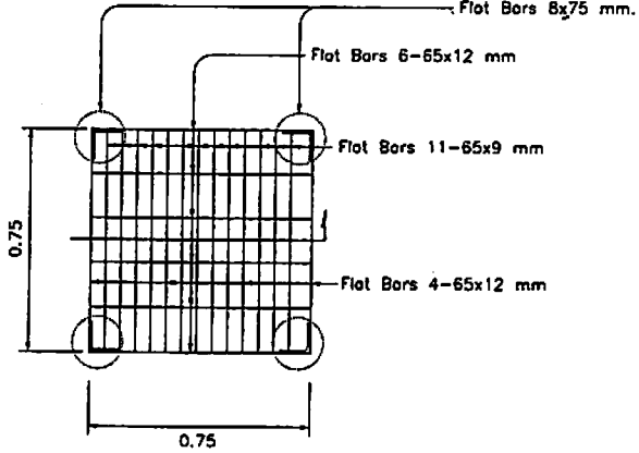
ขยายฝ้าตะแกรงเหล็ก 1:20
