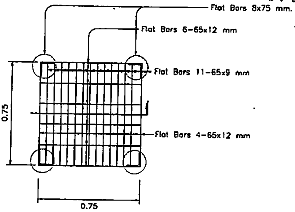
ขยายฟาดตะแกรงเหล็ก 1:20
