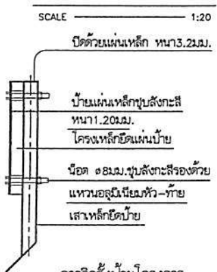
การติดตั้งบ้ายโครงการ
