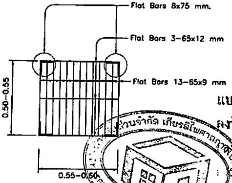
ขยายฟาดบ่อรับน้ำ 1:20
