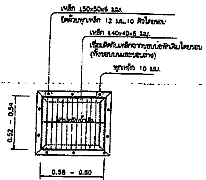
แปลนบ่อรับน้ำ 1:25
