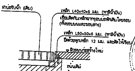
แปลนบ่อรับน้ำรูปตัดแบบปลั๊กดูข้าง เลขที่ ทน.อบ. 452/2567 ลงวันที่ 6 มี.ค. 2567
