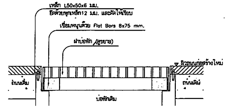
รูปตัด 1:10
