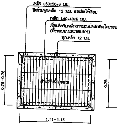
แบบส่นบ่อพัก 1:20
