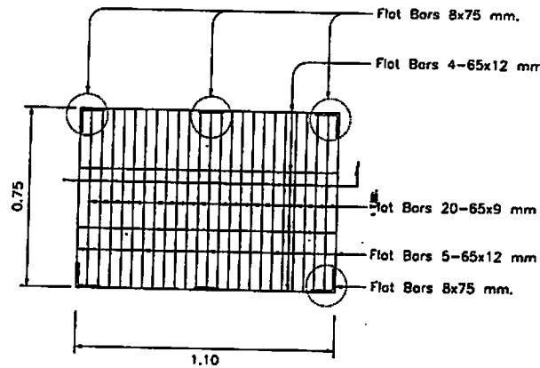
ขยายฝาตะแกรงเหล็ก 1:20
