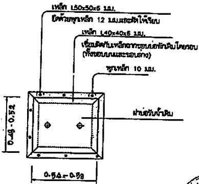
แบบส่นขอบน้ำ 1:20
