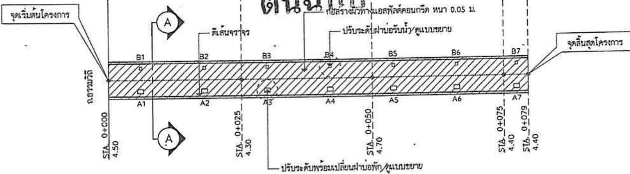
แปลนปูแอสฟัลต์คอนกรีต ดีไซน์จราจร SCALE 1:500
