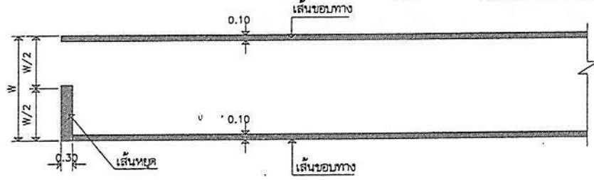
ขยายงานตีเส้นจราจร ไม่แสดงขนาดถาวร
