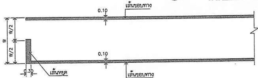
ขยายงานดีเส้นจราจร ไม่แสดงมาตราส่วน
