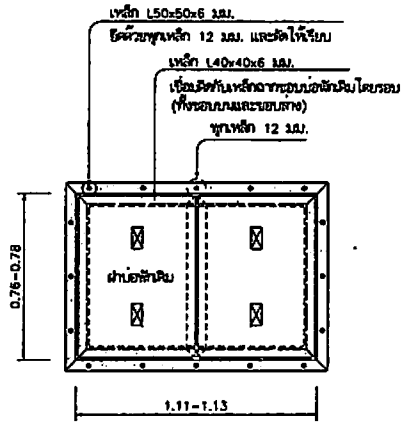
แปลนบ่อพัก 1:20
