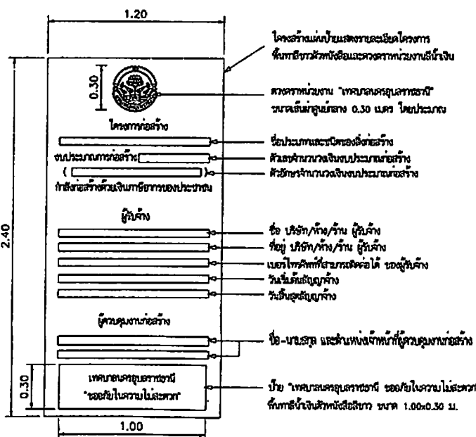
แผนผังรายละเอียดโครงสร้าง
