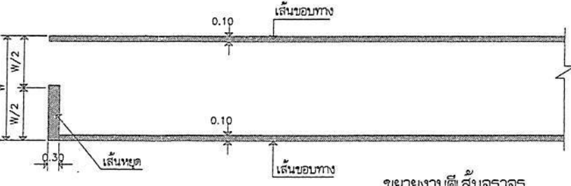
รูปตัด A-A non scale
