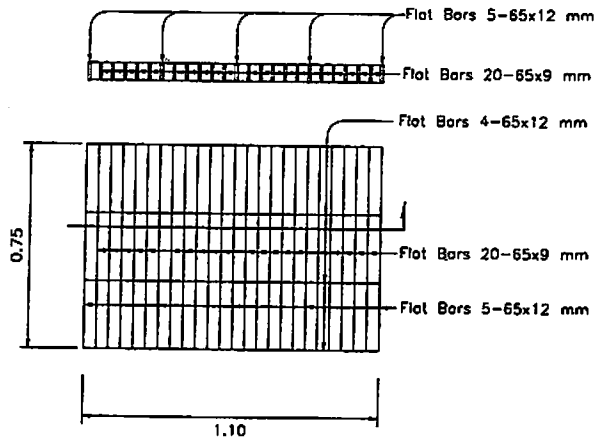
ขยายฝาอบอ้ากั้น 1:20
