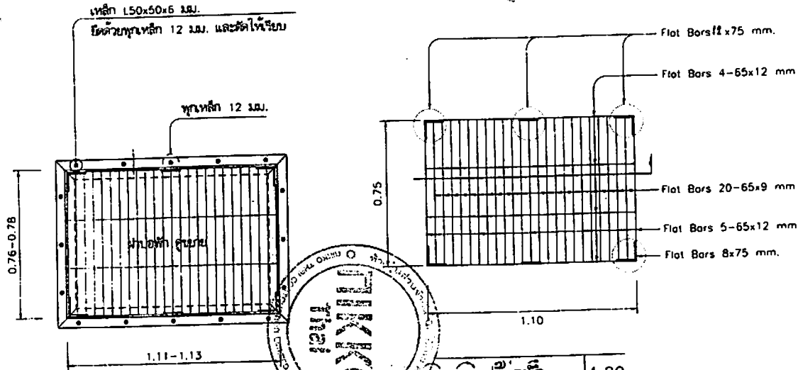
แปลนบ่อพัก 1:20
