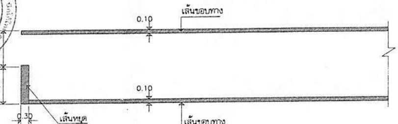
ขยายงานผิวเส้นจราจร ในขนาดมาตรฐาน
