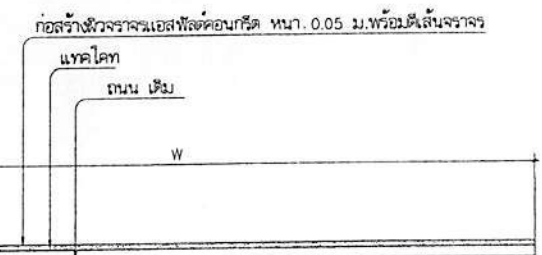
รูปตัด A-A non scale
