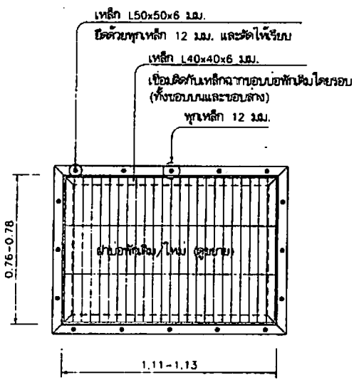
แปลนขอฟัก 1:20
