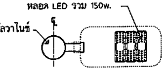
แบบขยาย B มาตราส่วน 1:20
