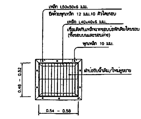
แปลนบ่อรับน้ำ 1:25
