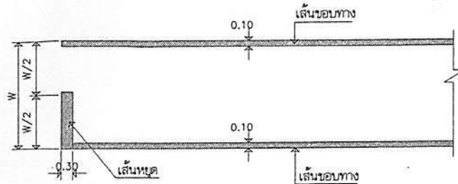
ขยายงานตีเส้นจราจร ในแอสฟัลท์คอนกรีต
