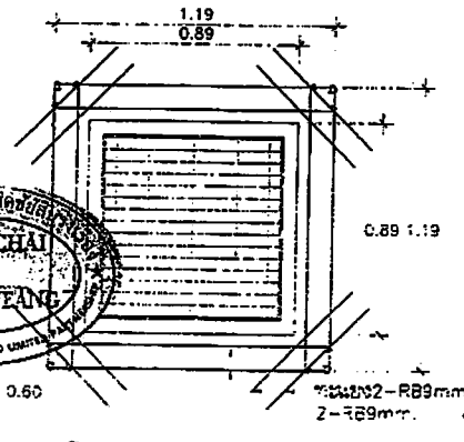
แบบขยายเหล็กเสริมรอบอ่ฟ้า SCALE 1:25
