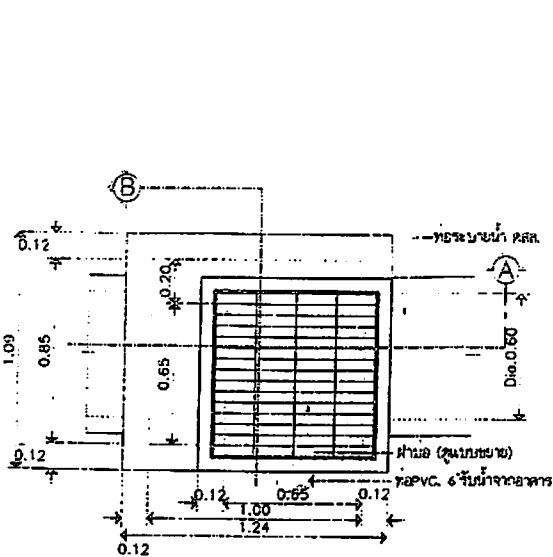
แปลนระบบระบายน้ำในผิวจราจร SCALE 1:25
