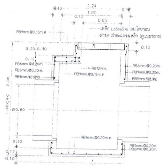
รูปตัด A-A SCALE 1:25
