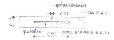
CONTRACTION JOINT 1:20 (ทุกระยะ 6.00 ม.)
