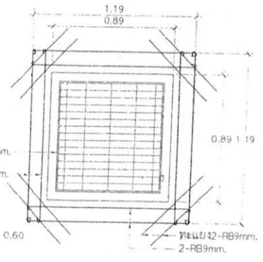
แบบขยายเหล็กเสริมรอบอพัก SCALE 1:25
