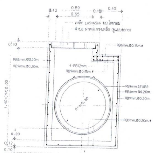
รูปตัด B-B SCALE 1:25
