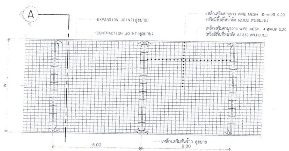
แปลนถนน ค.ส.ล. (หนา 0.15 ม.) SCALE 1:100
