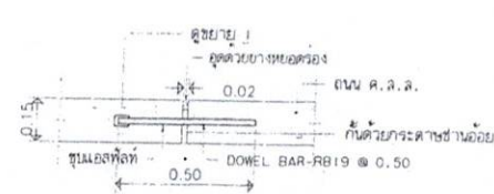
EXPANSION JOINT 1:20 (ทุกระยะไม่เกิน 60.00 ม.)
