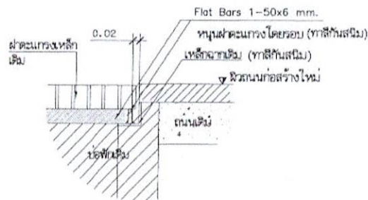
รูปตัด 1 1:10
