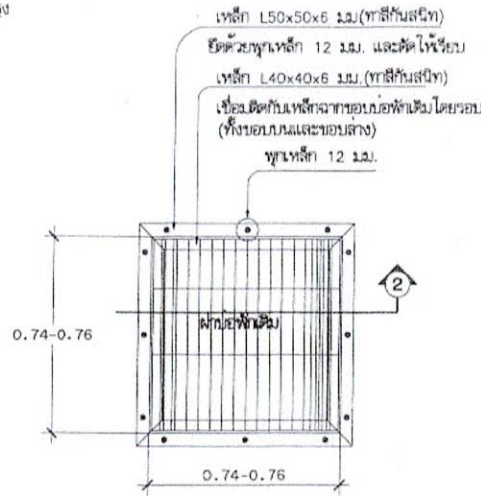
แบบสอยกผ้าอพัก (B)
