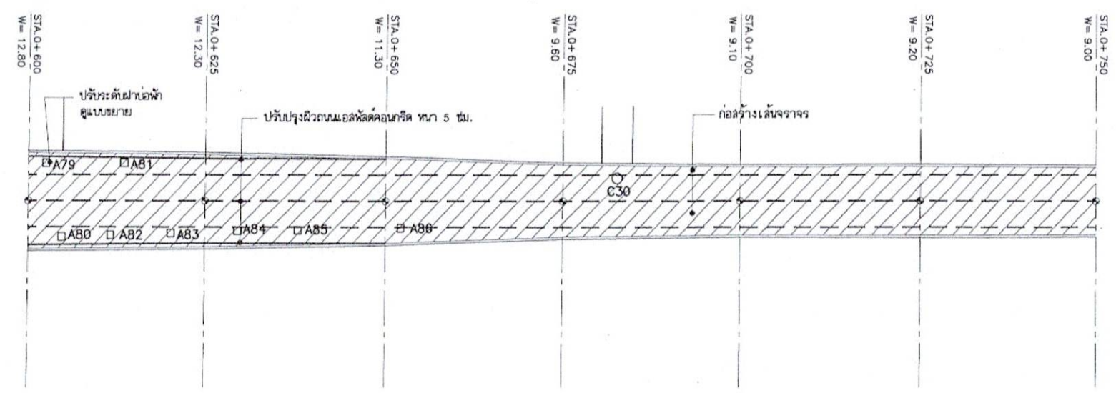
แผนปรับปรุงผิวทางแอสฟัลต์คอนกรีต ถนนพโลชัย SCALE 1 : 500 (ช่วงถนนช่วงนอก-ซอยจรจรัญ 11)
