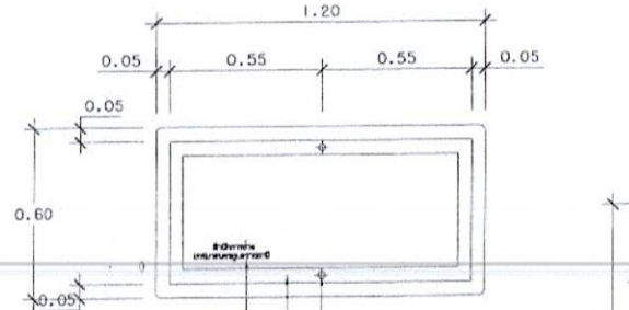
บ้ายโครงการงานก่อสร้าง SCALE 1:20
