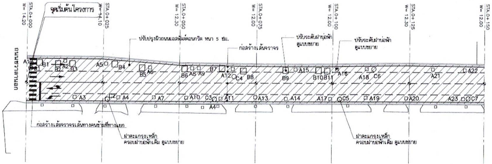
แปลนปรับปรุงผิวทางแอสฟัลต์คอนกรีต ถนนพหลโยธย์ SCALE 1:500 (ช่วงถนนชวาลานอก-ซอยจรรยาสิทธิ์ 11)
