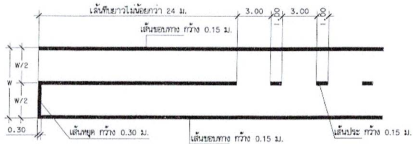
ขยายงานตีเส้นจราจร
