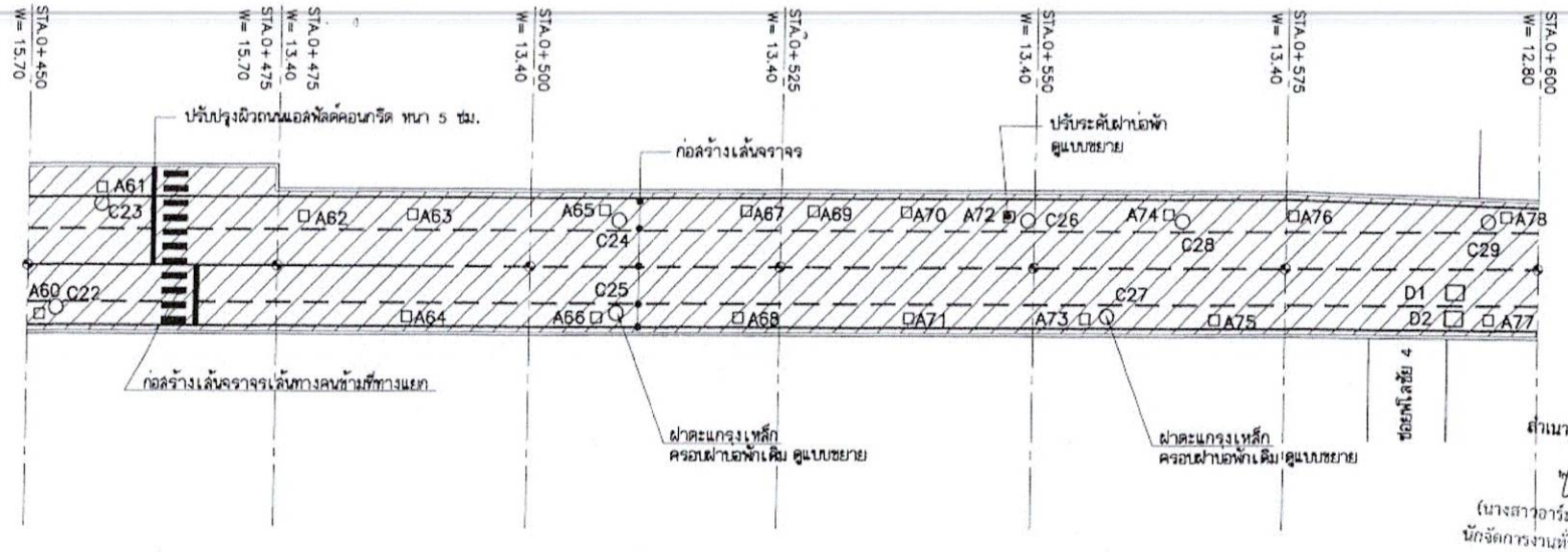
แปลนปรับปรุงผิวทางแอลพีดีคอนกรีต ถนนพิไลชัย SCALE : 1 : 500 (ช่วงถนนชวาลานอก-ซอยจรัลพิชัย 11) H I U O N
