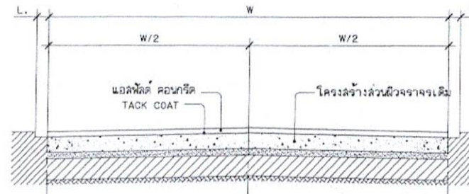
รูปตัดถนน มาตราส่วน 1:25
