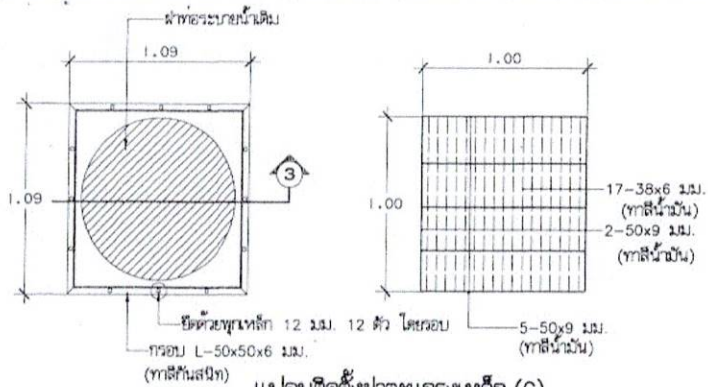
แปลนติดตั้งฟาดะแครงเหล็ก (C)
