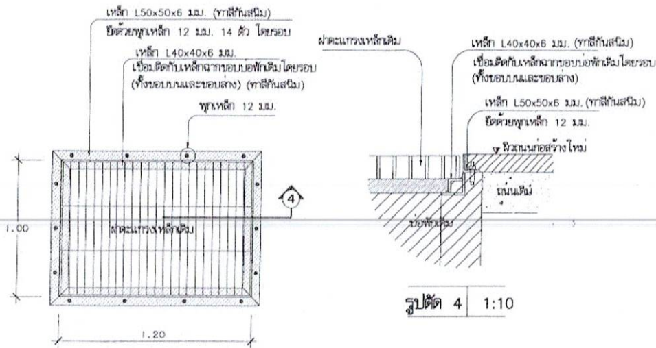
แปลนยกฟาดบ่อพัก (D)
