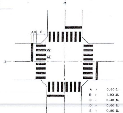
มาตรฐานเส้นทางคนข้ามที่ทางแยก SCALE no.
