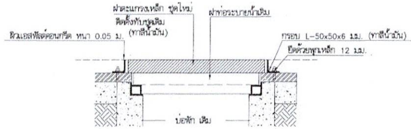
รูปตัด 3
