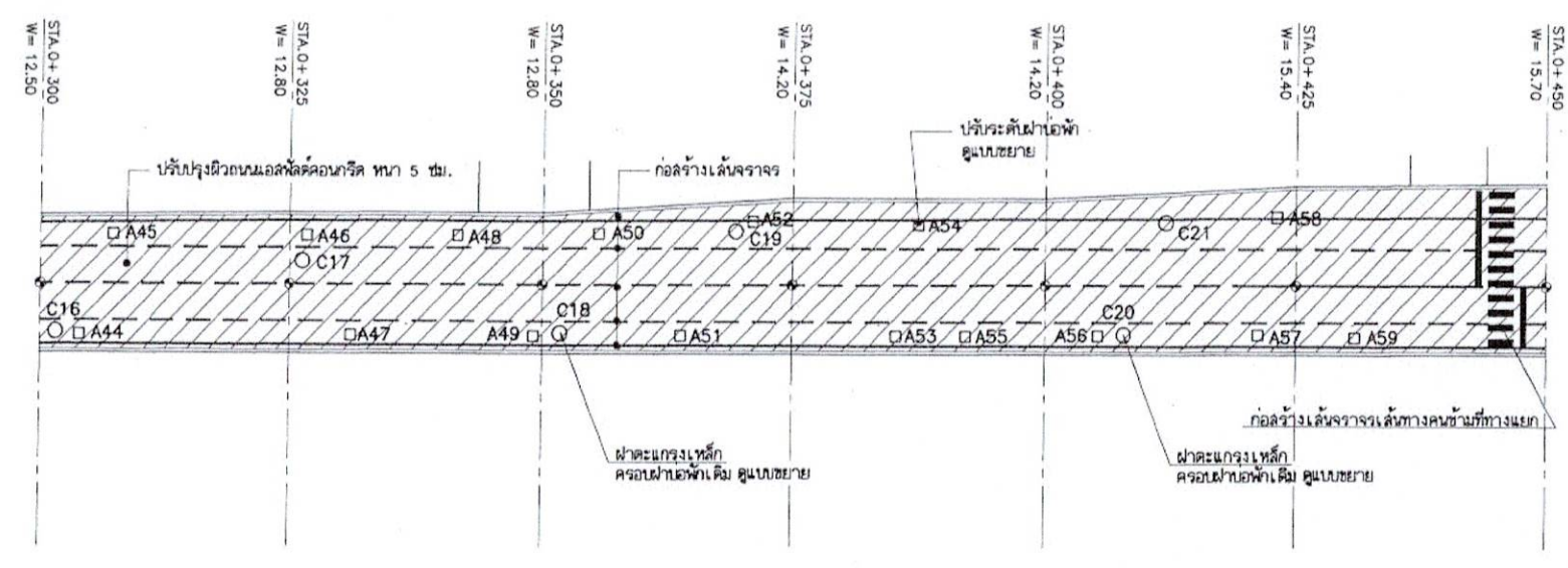
แปลนปรับปรุงผิวทางแอลพีดีคอนกรีต ถนนพิไลชัย SCALE : 1 : 500 (ช่วงถนนชวาลานอก-ซอยจรัลพิชัย 11) H I U O N
