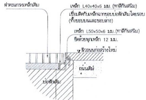
รูปตัด 2 1:10
