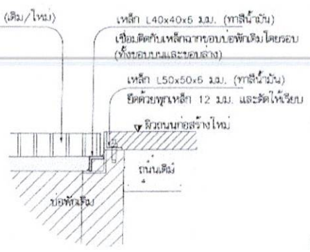
รูปตัด 1:10
