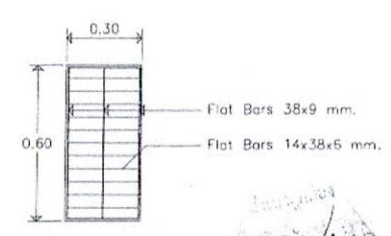
แบบผ้าบ่อพัก มติครุฑวง 1:20
