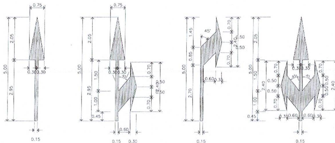
มาตรฐานเครื่องหมายลูกศรบนผิวทาง
