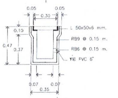
แบบขยายบ่อพัก D มติครุฑวง 1:20
