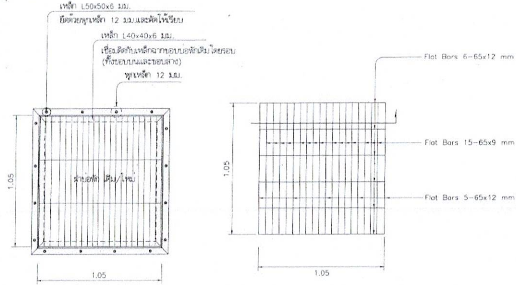
แปลนบ่อพัก 1:20
