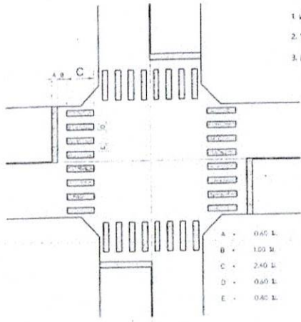
มาตรฐานเส้นทางคนข้ามที่ทางแยก
