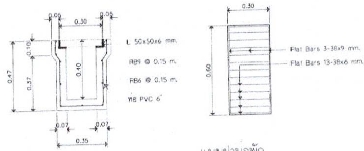
แบบฝาบ่อพัก มาตราส่วน 1:20
