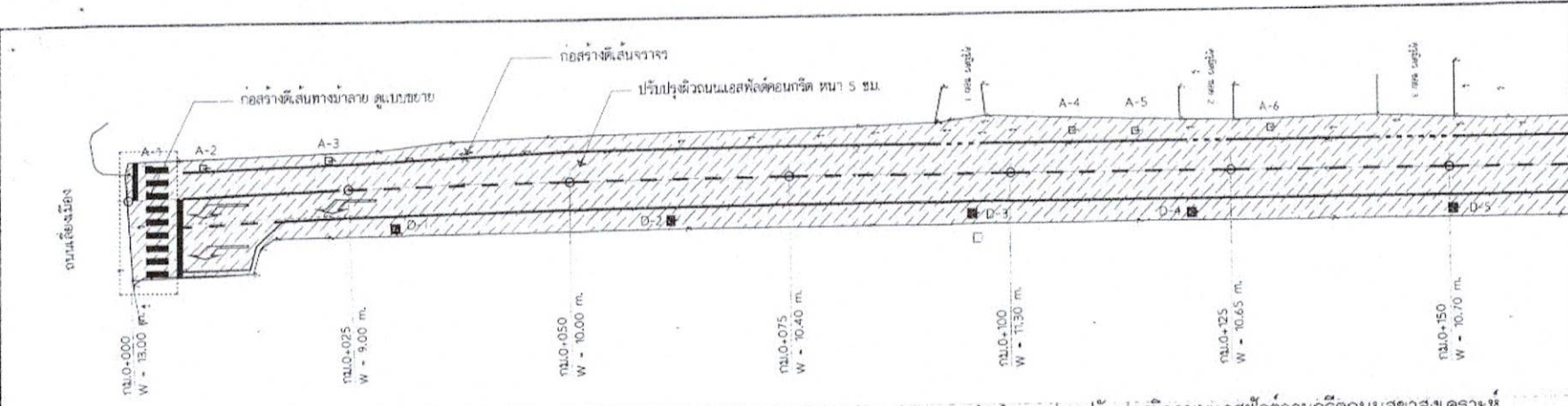
ดินเหนียว ↕ แปลนปรับปรุงผิวถนนแอสฟัลต์คอนกรีตถนนลูกรังสายวงแหวน ช่วงถนนชยางกูร - ซอยชยางกูร 12.3 มาตราส่วน 1:500
