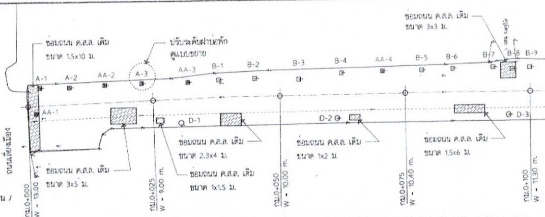
ดินเหนียว แปลนแสดงตำแหน่งขอมแซมถนน ค.ส.ล. เดิมและปรับระดับฝ้าบ่อพักเดิม ถนนสุขุมวิท (ช่วงถนนขยายทาง - ซอยขยายทาง 12.3) ขนาดกระดาษ 1500
