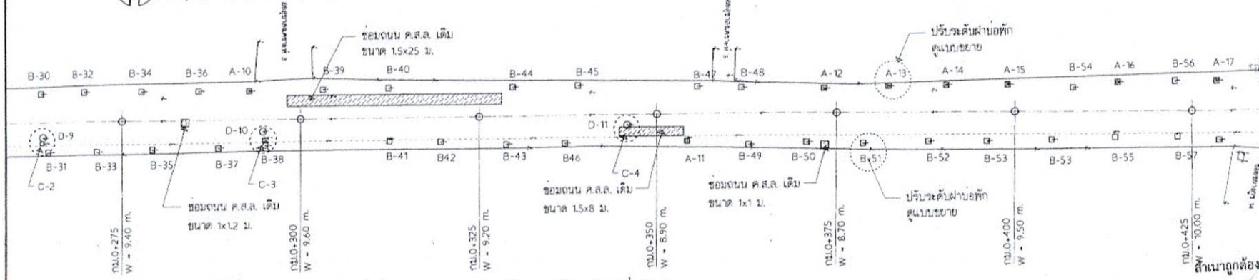
ดินเหนียว แปลนแสดงตำแหน่งขอมแซมถนน ค.ส.ล. เดิมและปรับระดับฝ้าบ่อพักเดิม ถนนสุขุมวิท (ช่วงถนนขยายทาง - ซอยขยายทาง 12.3) ขนาดกระดาษ 1500
