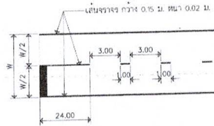
มาตรฐานเส้นแบ่งช่องจราจร
