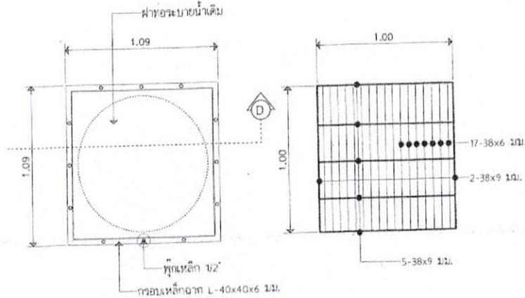
แบบขยายฝาบ่อพัก D มาตราส่วน 1:25
