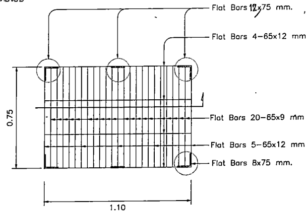
ขยายฝาอ่พัก 1:20
