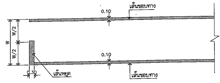
ขยายงานตีเส้นจราจร ไม่แสดงมาตราส่วน
