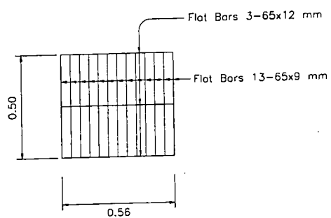
ขยายฝาบ่อรับน้ำ 1:20
