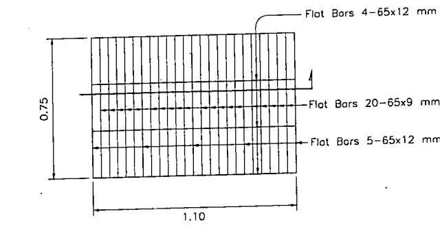
ขยายฝาบ่อพัก 1:20
