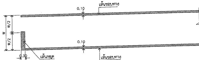
ขยายงานตีเส้นจราจร ไม่แสดงขนาดบางส่วน
