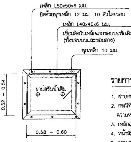
แปลนบ่อรับน้ำ 1:20
