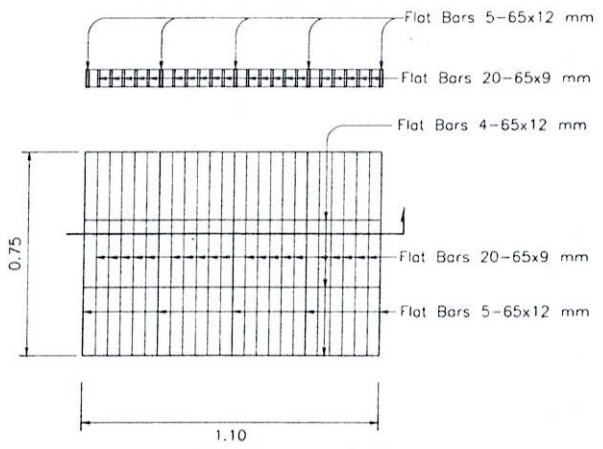
ขยายฝายบ่อพัก 1:20
