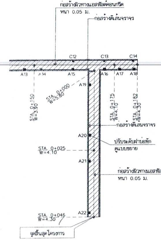
แปลนแปลนแอสฟัลต์คอนกรีต ตีเส้นจราจร
