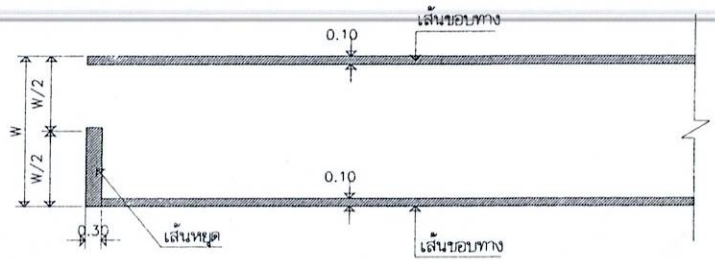
รูปตัด 1:10
