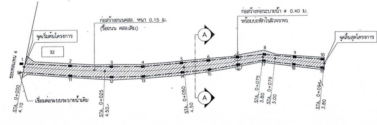
แปลนก่อสร้างถนน ค.ส.ล. พร้อมท่อระบายน้ำ ซอยพลพเนน 6 (ข้างบ้านเลขที่ 32) มาตราส่วน 1:500 ทิศเหนือ
