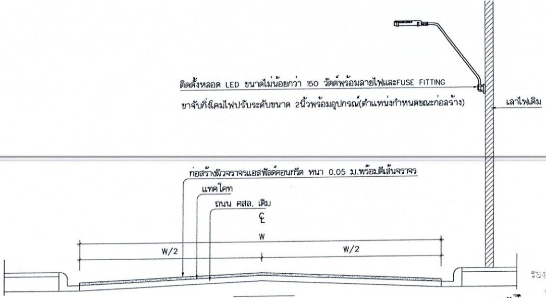
รูปตัด A-A non scale
