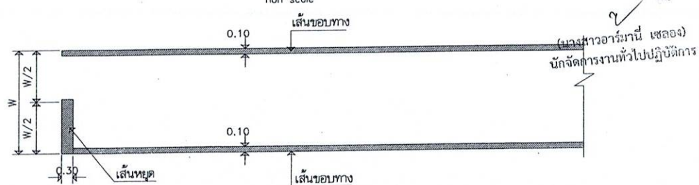
ขยายงานตีเส้นจราจร
