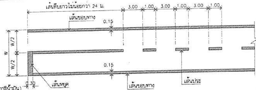
ขยายงานที่เส้นจราจร ไม่แสดงขนาดส่วน
