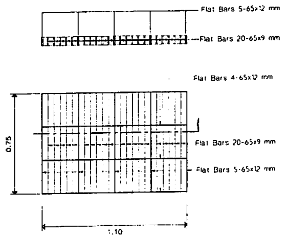
แบบขยายฝายอพัทัก B ขนาดฐาน 120
