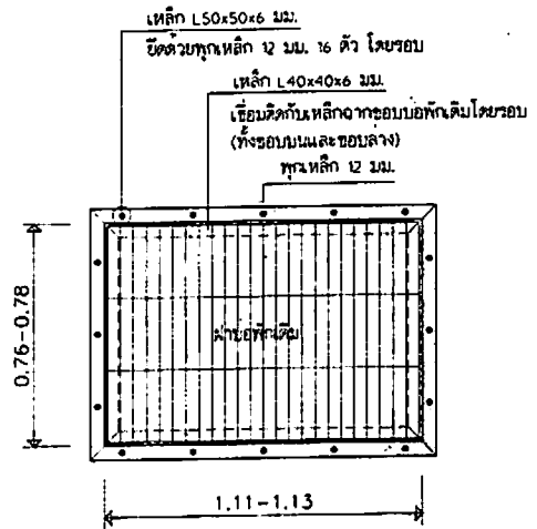
แปลนฝายอพัทัก A ขนาดฐาน 120
