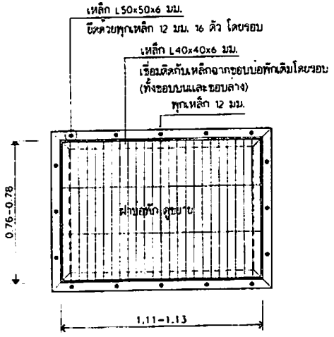
แปลนฝายอพัทัก B ขนาดฐาน 120
