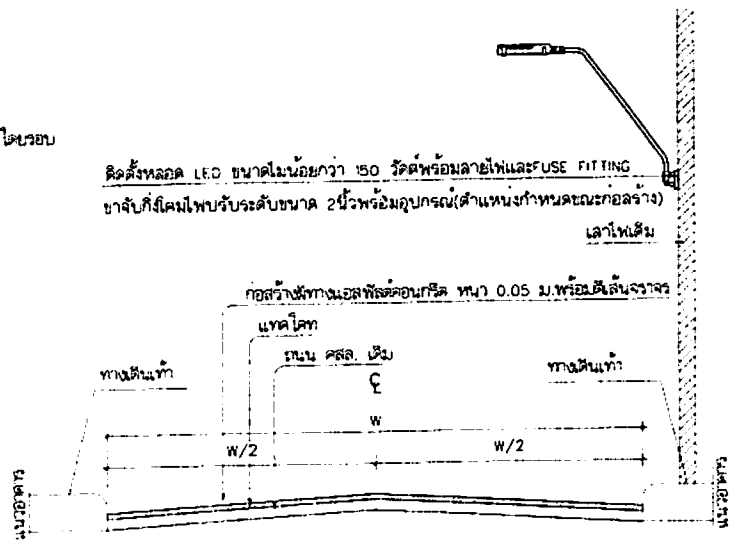
รูปตัด A-A not scale
