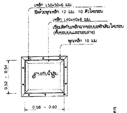
แปลนบ่อปรับน้ำ F 1:20
