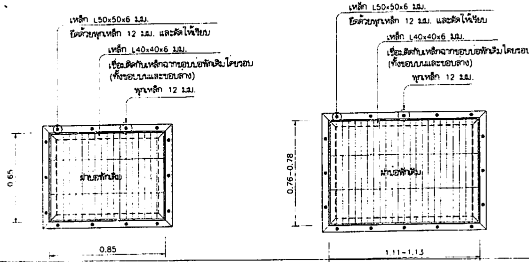
แปลนบ่อพัก A 1:20
