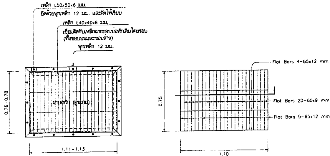
ขยายฝับบ่อพัก B 1:20
