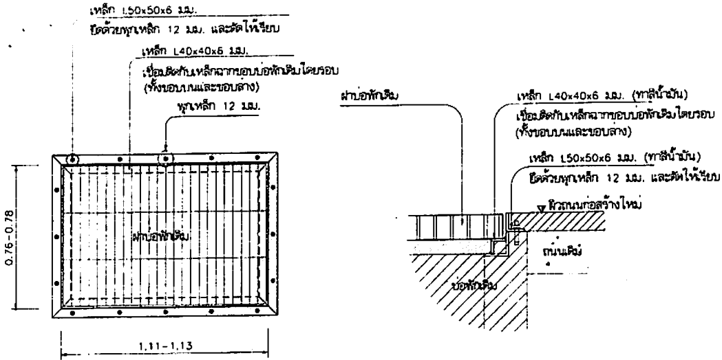
รูปตัด 1:10
