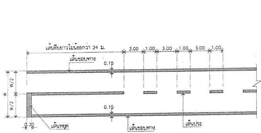
ขยายงานตีเส้นจราจร ไม่แสดงขนาดถาวร
