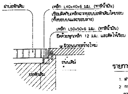
รูปตัด 1:10
