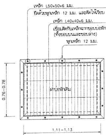
แปลนบ่อพัก B 1:20
