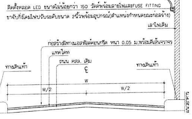
รูปตัด A-A non scale
