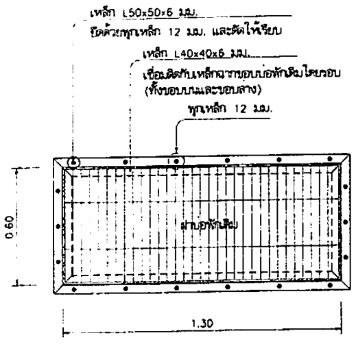
แปลนบ่อพัก D 1:20
