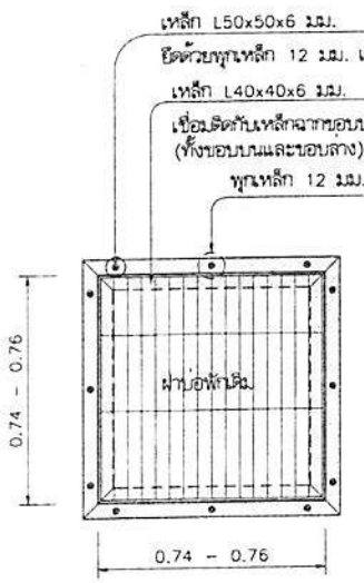
แปลนบ่อพัก A 1:20
