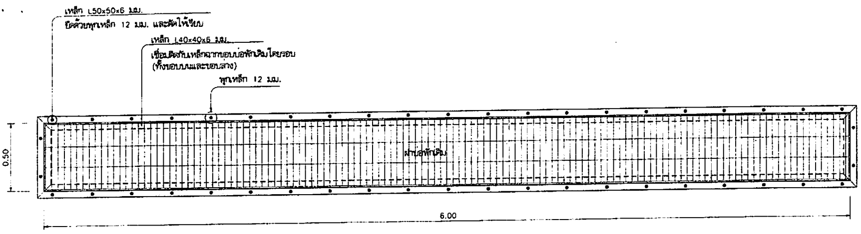
แปลนบ่อพัก C 1:20
