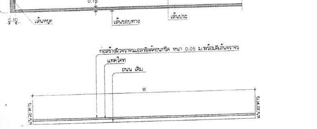
รูปตัด A-A non scale
