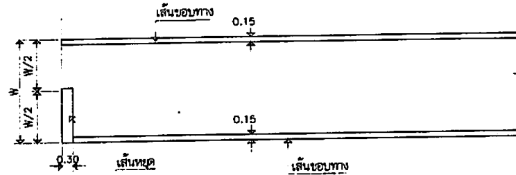
ขยายงานติดตั้งเส้นจรรยา ในเขตเทศบาลส่วน
