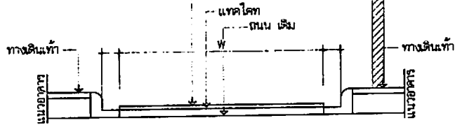
รูปตัดถนน ในเขตเทศบาล
