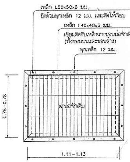
แปลนบ่อพัก A 1:20
