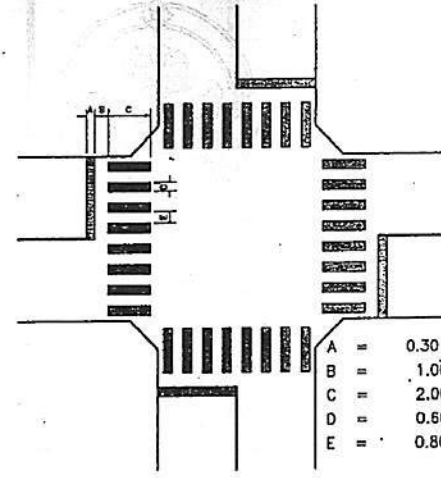
มาตรฐานเส้นทางคนข้ามที่ทางแยก
