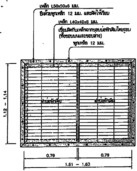
แปลนบ่อพัก E / 1:20
