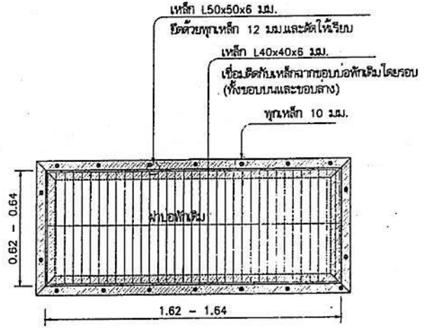
แปลนบ่อพัก C / 1:25
