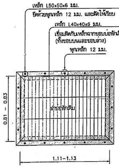
แปลนบ่อพัก A / 1:20
