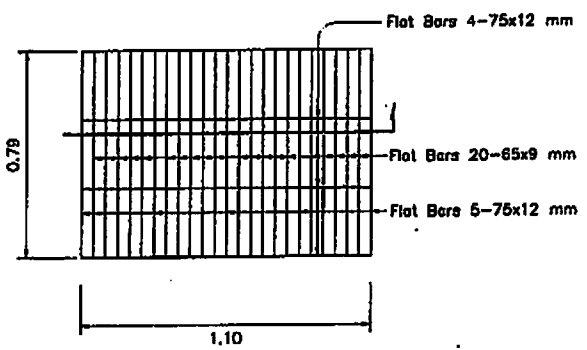
ขยายฝ้าบ่อพัก B 1:20
