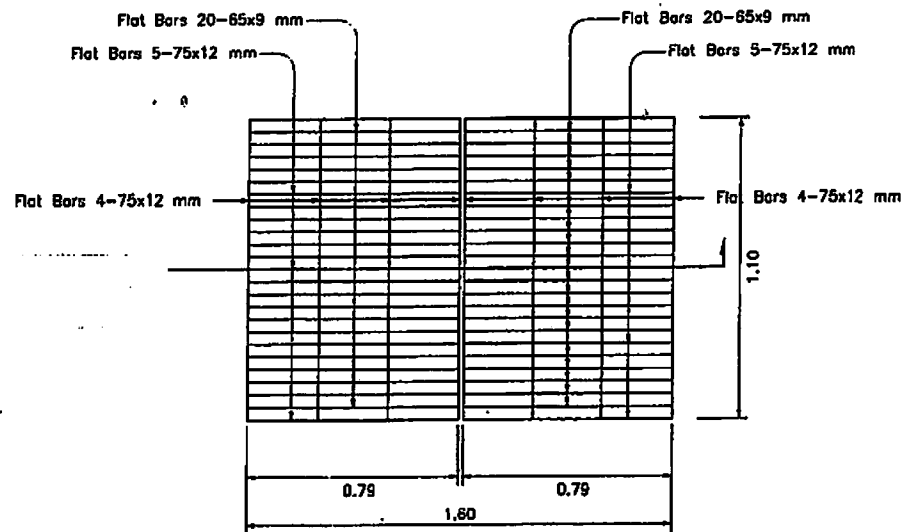
ขยายผ่านบ่อพัก F 1:20
