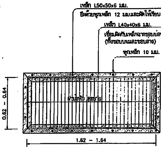
แปลนบ่อพัก D 1:25
