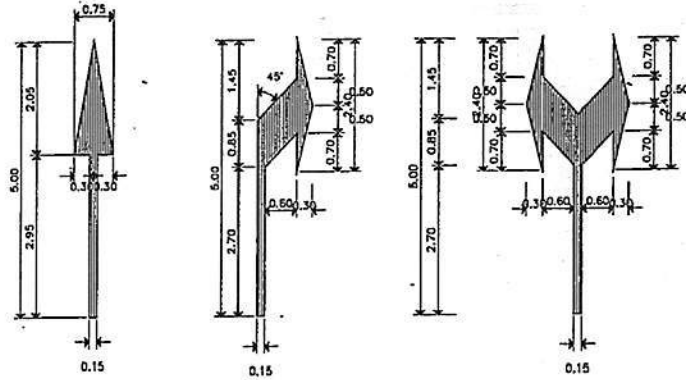
มาตรฐานเครื่องหมายลูกศรบนหัวทาง
