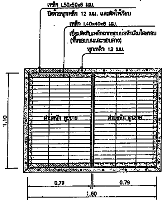
แปลนบ่อพัก F 1:20
