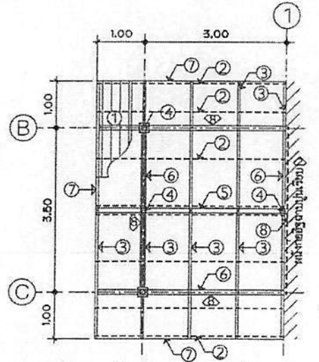
แปลนโครงสร้างหลังคา มุมทางเข้า (ปรับปรุง) มาตราส่วน 1:75
