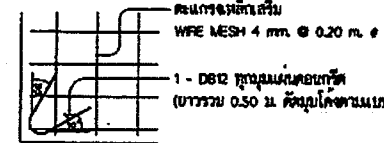
ขยาบการเสริมเหล็กกันจ้าว
