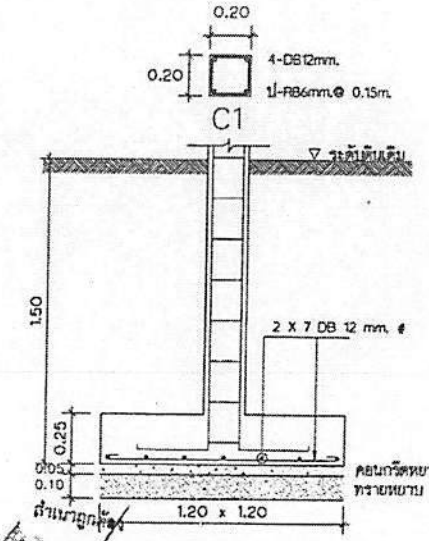
รูปตัดฐานราก F1
