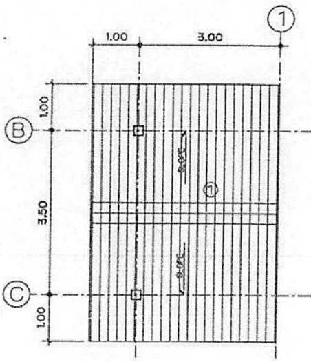
แปลนสร้างหลังคา มุมทางเข้า (ปรับปรุง) มาตราส่วน 1:75
