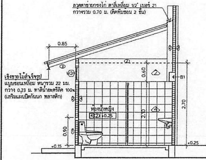
รูปตัดห้องน้ำ - ส้วม (สร้างใหม่)
