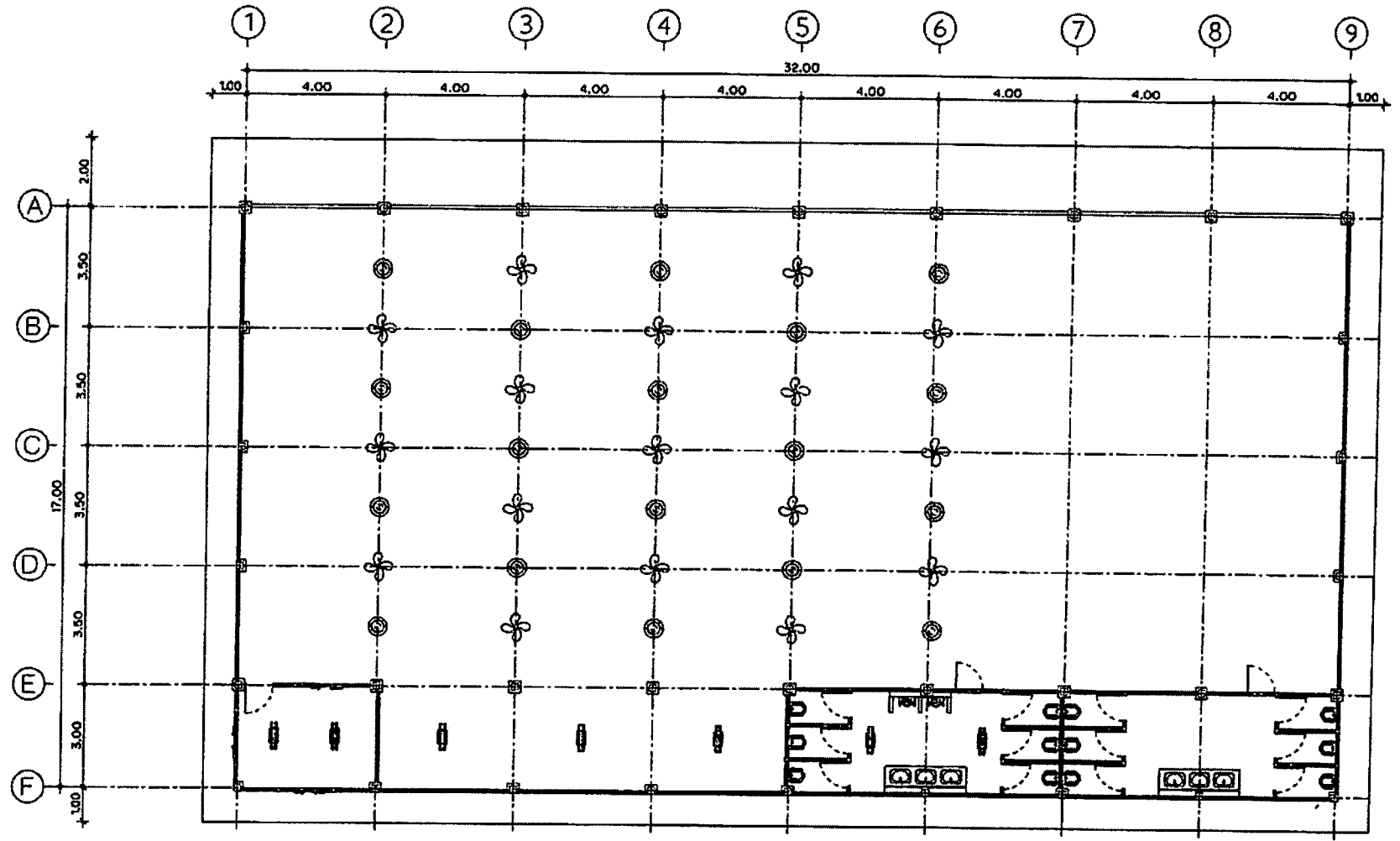
แปลนไฟฟ้า (เดิม) : ร้อยถอน มาตราส่วน 1 : 125
