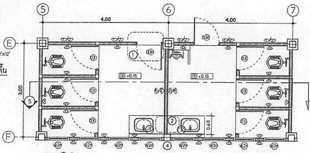
ขยายแปลนห้องน้ำ - ส้วม (ปรับปรุง)
