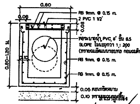
ขยาบข้อพัก คสล. MH ก่อสร้าง @ ไม่เกิน 12 ม.
