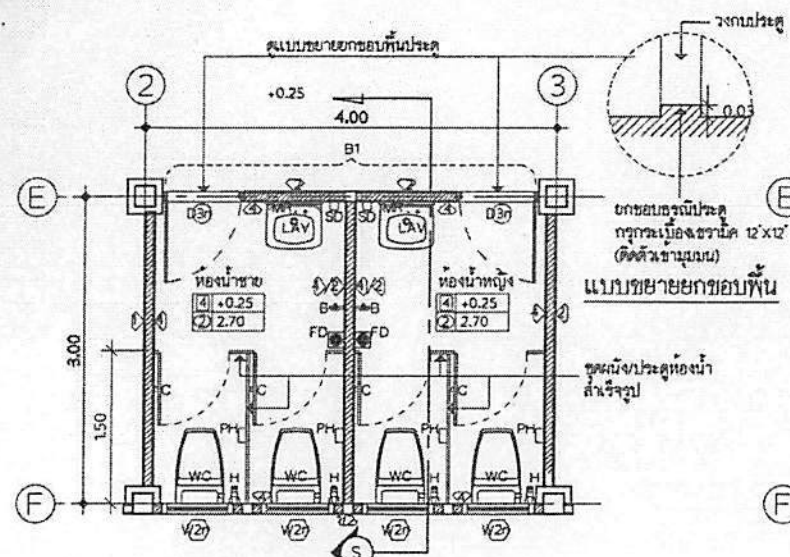
ขยายแปลนห้องน้ำ - ส้วม (สร้างใหม่)
