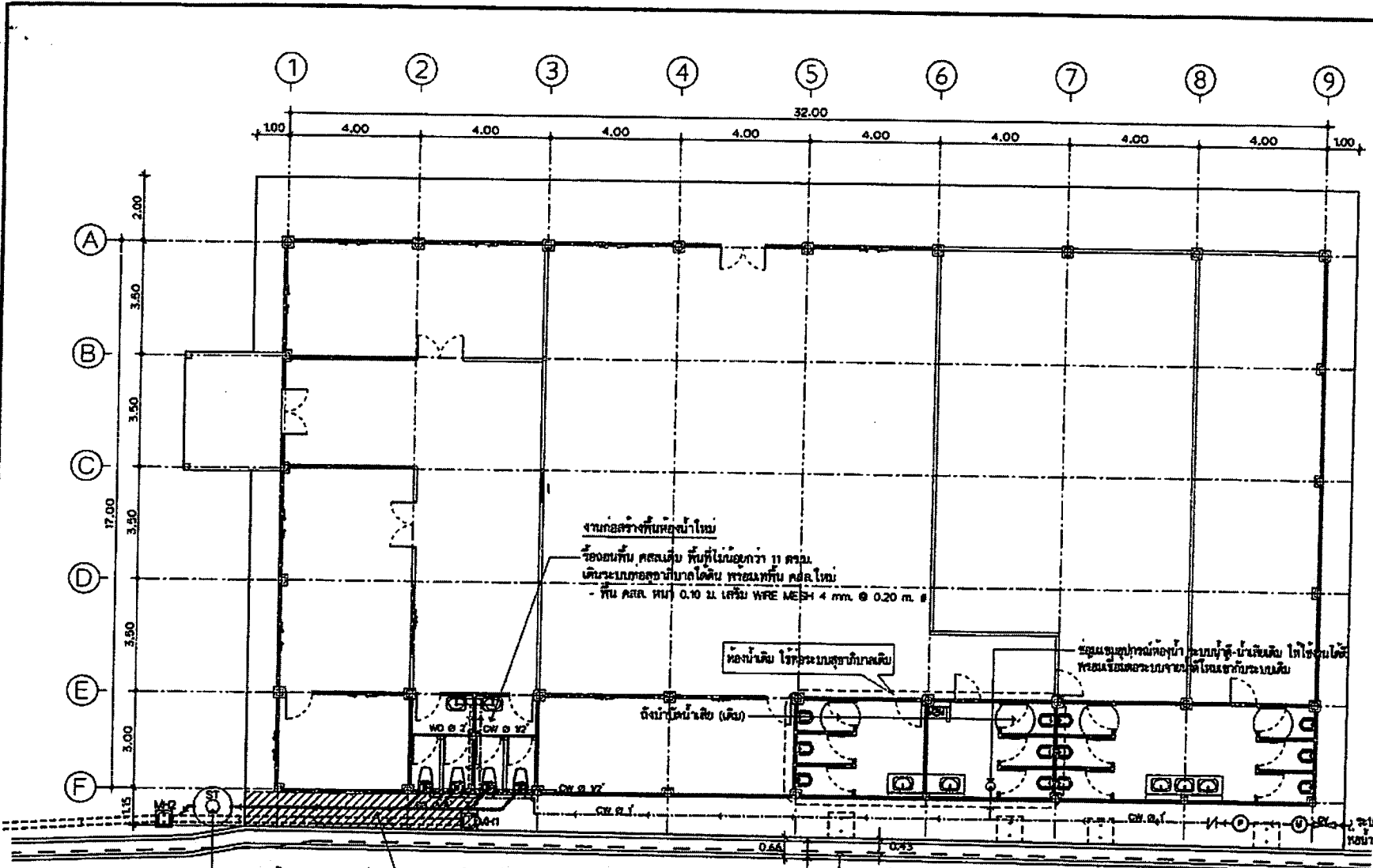
แบบระบบสุขาภิบาล มาตราส่วน 1 : 125
