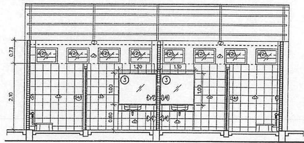
รูปตัดห้องน้ำ - ส้วม (ปรับปรุง)
