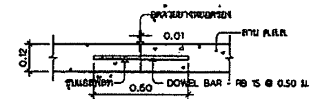
CONTRACTION JOINT (ระยะห่างไม่เกิน 5.00x0.00 ม.)
