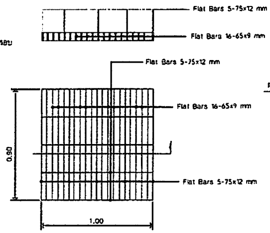
แบบขยายฝ้ายอพัก F มาตราส่วน 1:20
