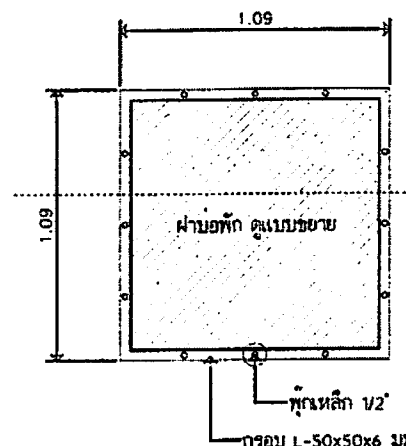
แปลนฝายอพัก D ขนาดส่วน 1:20
