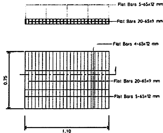
แบบขยายฝานอพัก A ขนาดส่วน ๓20
