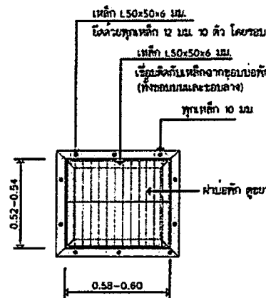
แปลนฝานอพัก C ขนาดส่วน ๓20
