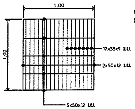
แบบขยายฝายอพัก D ขนาดส่วน 1:20
