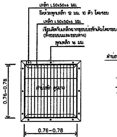
แบบขยายฝานอพัก B ขนาดส่วน ๓20
