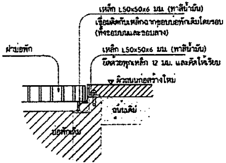
รูปตัดฝายอพัก E ไม่แสดงขนาดส่วน
