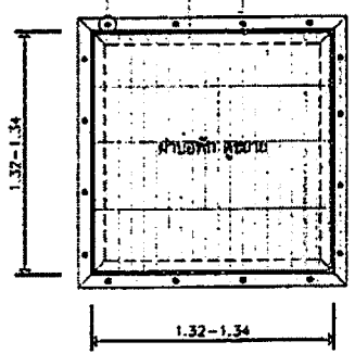
แปลนฝายอพัก E ขนาดส่วน 1:20
