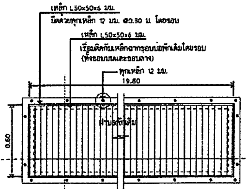
แปลนบ่อพัก H มาตราส่วน 1:20
