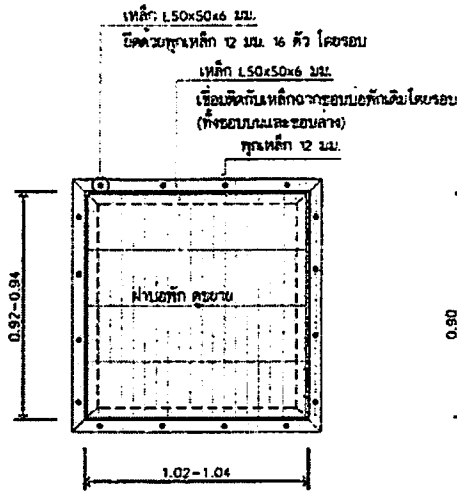
แปลนฝ้ายอพัก F มาตราส่วน 1:20
