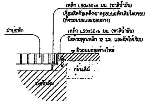
รูปตัดบ่อพัก H ไม่แสดงมาตราส่วน
