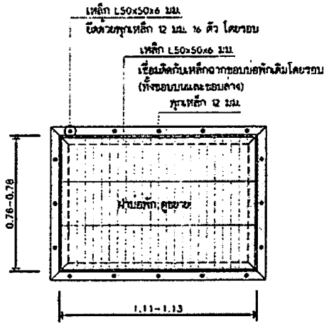
แปลนฝานอพัก A ขนาดส่วน ๓20
