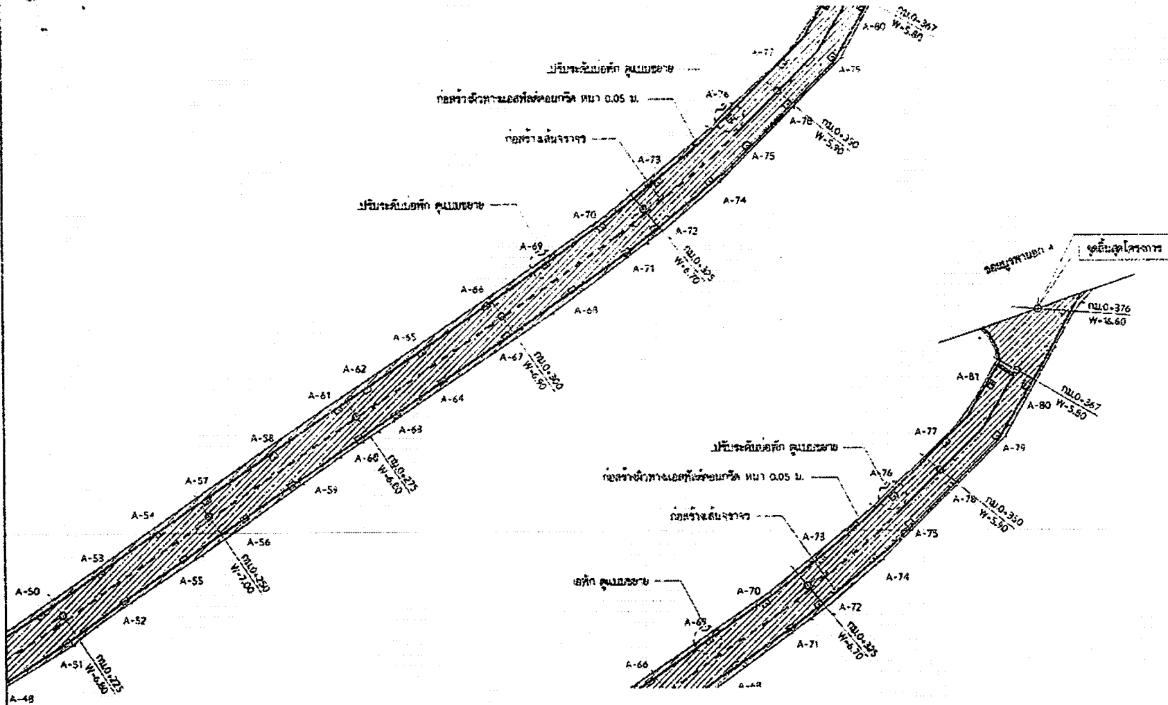
แบบแปลนปรับปรุงผิวทางแอสฟัลต์คอนกรีต ขอบเขตงานนอก 2 มาตราส่วน 1:500
