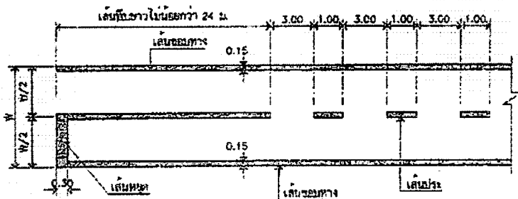
ขยายงานตีเส้นจราจร ไม่ลงขนาดตาม
