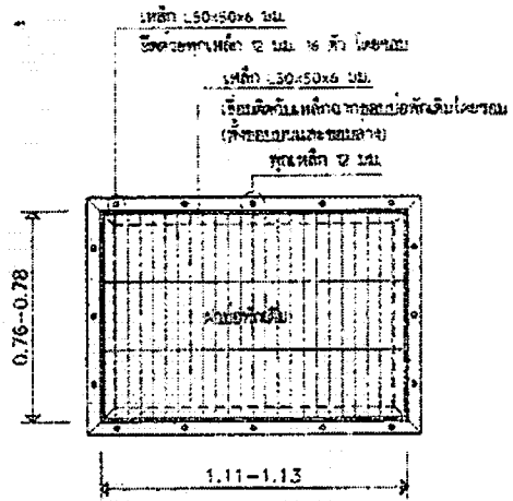
แบบขยายฝ้ายอก A มาตราส่วน 1:20
