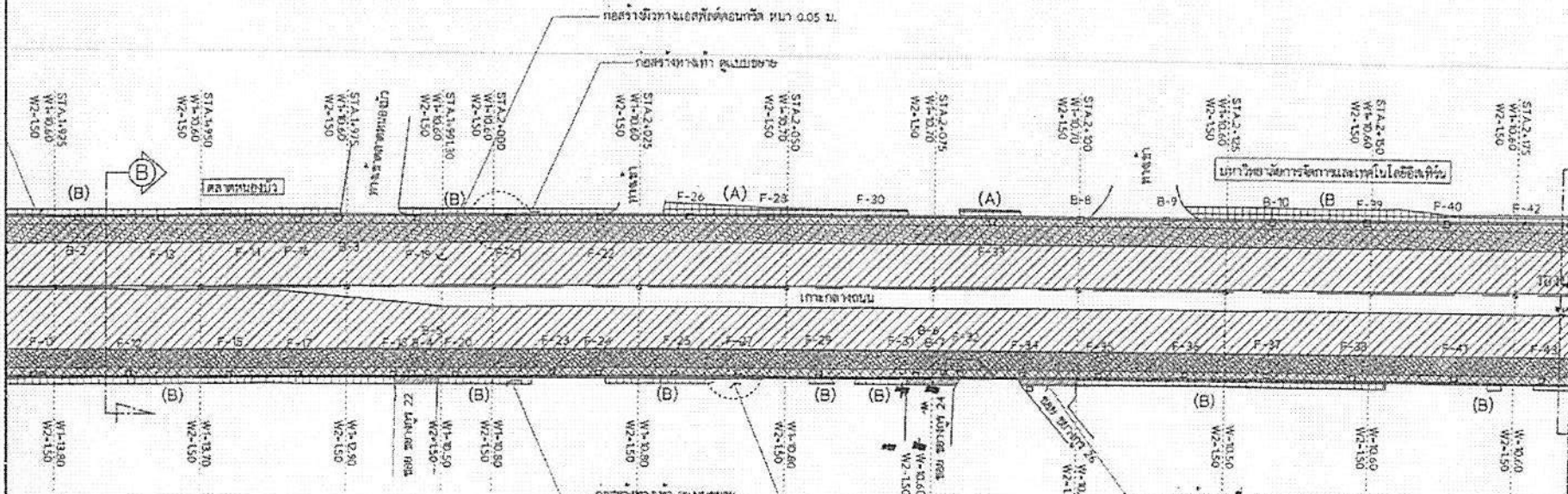
แปลนปรับปรุงถนนแอสฟัลต์คอนกรีต มาตราส่วน 1:750
