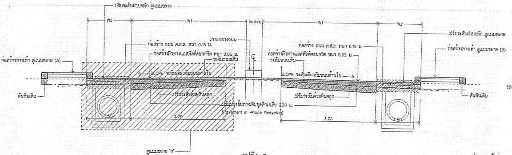
รูปตัด C มาตราส่วน 1:25
