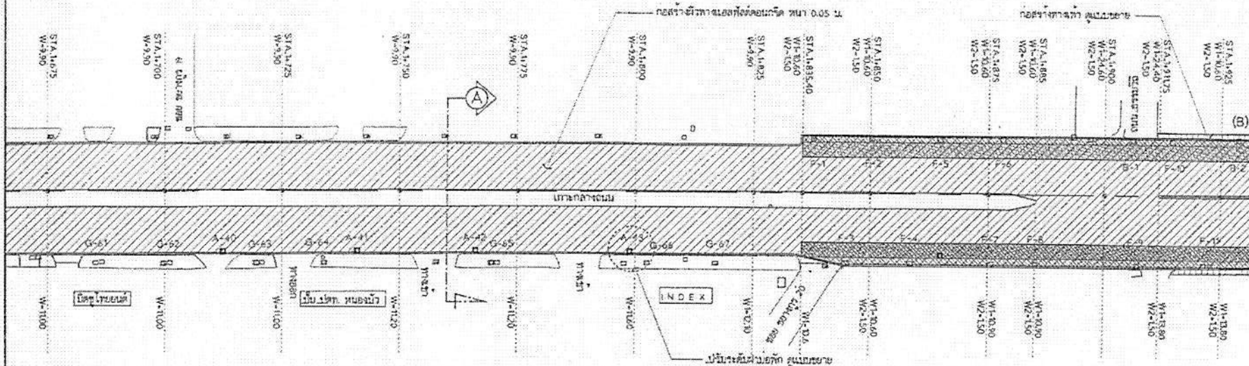
แปลนปรับปรุงถนนแอสฟัลต์คอนกรีต มาตราส่วน 1:750
