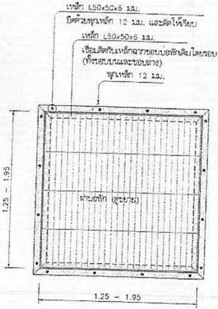
แปลนบ่อพัก A 1:20
