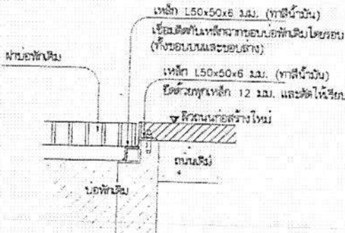
รูปตัด 1:10
