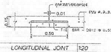
CONTRACTION JOINT 1:20 (ขนาด 6.00 ม.)
