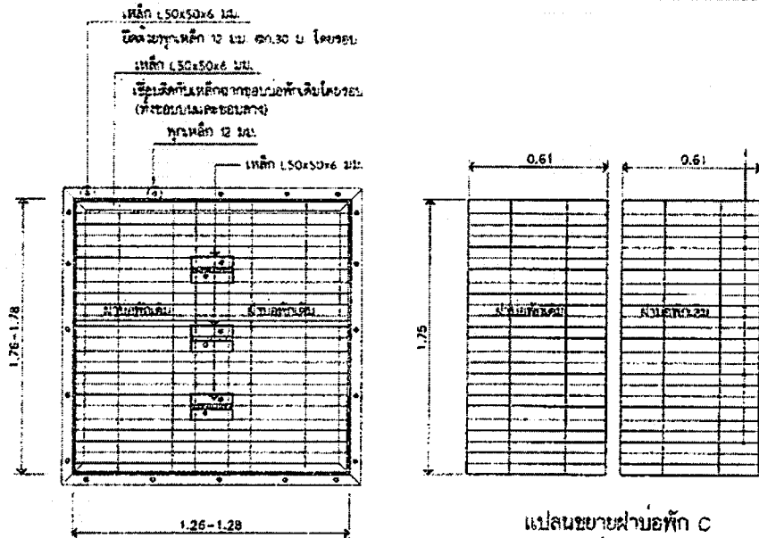
แปลนฝ้าบ่อพัก C ขนาดฐาน 120
