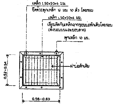
แปลนฝ้าบ่อพัก E ขนาดฐาน 120
