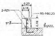
ขยายคันทัน ค.ส.ล. มาตราส่วน 1:25
