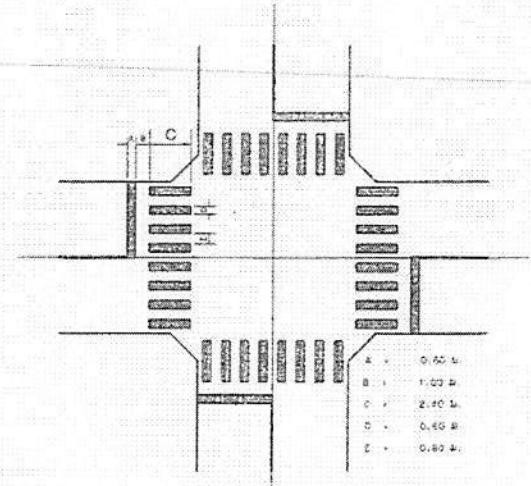
มาตรฐานเส้นทางคนข้ามที่ทางแยก SCALE 1:200
