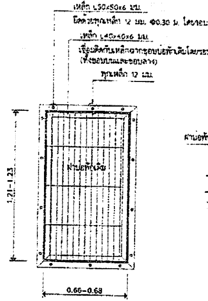
แปลนฝ้าบ่อพัก D ขนาดหน้ากว้าง ๖๖
