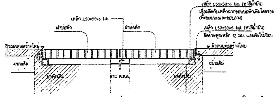
รูปตัดฝ้าบ่อพัก L ไม่แสดงขนาดหน้ากว้าง
