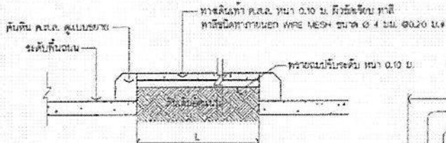
รูปตัดขยายทางเท้า ค.ส.ล. Scale 1 : 25
