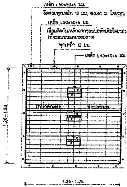
แปลนฝ้าบ่อพัก B ขนาดหน้ากว้าง ๖๖
