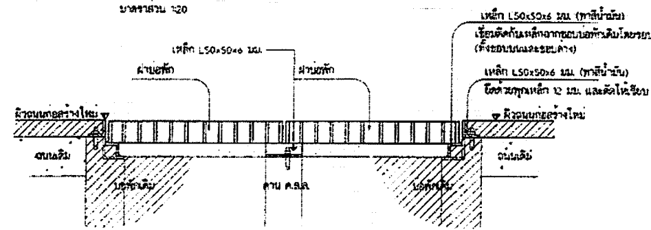
รูปตัดฝ้าบ่อพัก C ไม่แสดงขนาดฐาน
