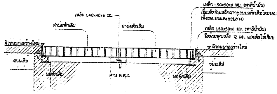
รูปตัดฝ้าบ่อพัก B ไม่แสดงขนาดหน้ากว้าง
