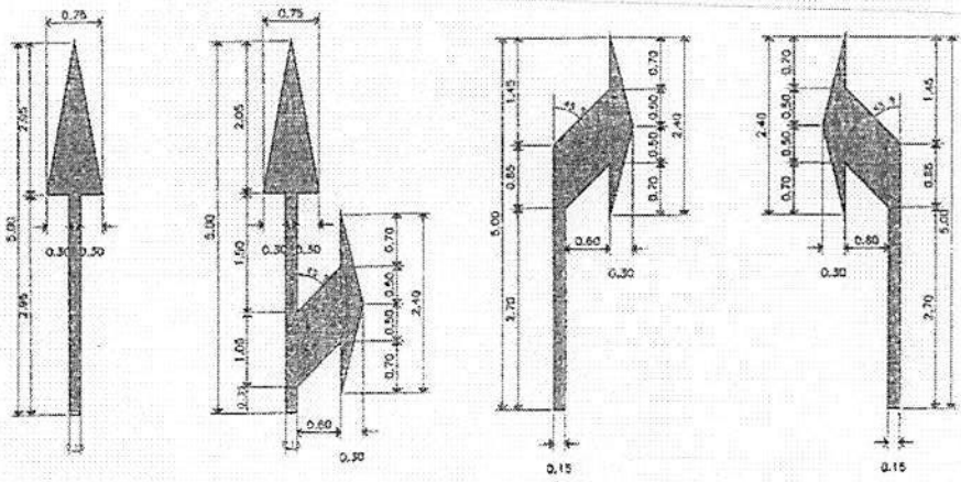
มาตรฐานเครื่องหมายลูกศรวงเวียนทาง SCALE 1:50
