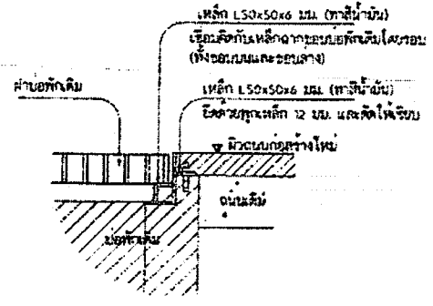
รูปตัดฝ้าบ่อพัก E ไม่แสดงขนาดฐาน
