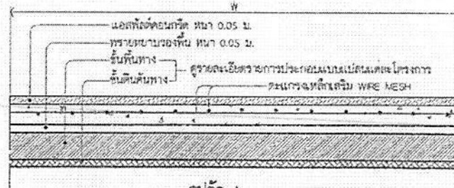
รูปตัด A SCALE 1:25
