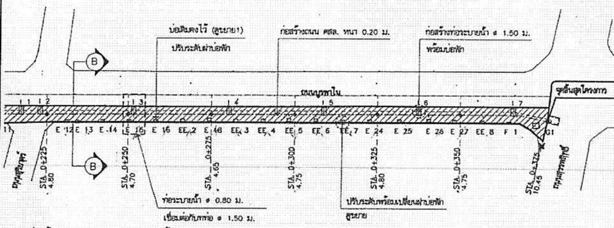
แปลนก่อสร้างถนน ค.ส.ล.และระบอบระบายน้ำ
