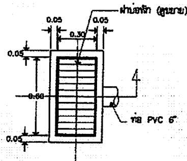
ขยายฝาท่อชักหน้า H SCALE 1:20
