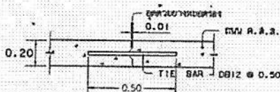
LONGITUDINAL JOINT 1:20
