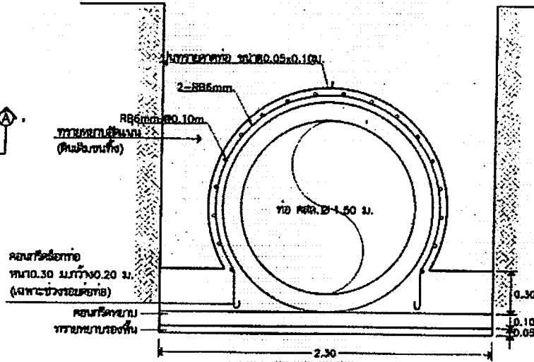
รูปตัดท้อระบายน้ำ SCALE 1:25
