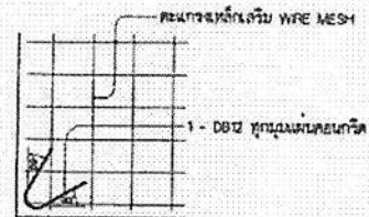
ขยายการเสริมเหล็กกับราว SCALE 1:50
