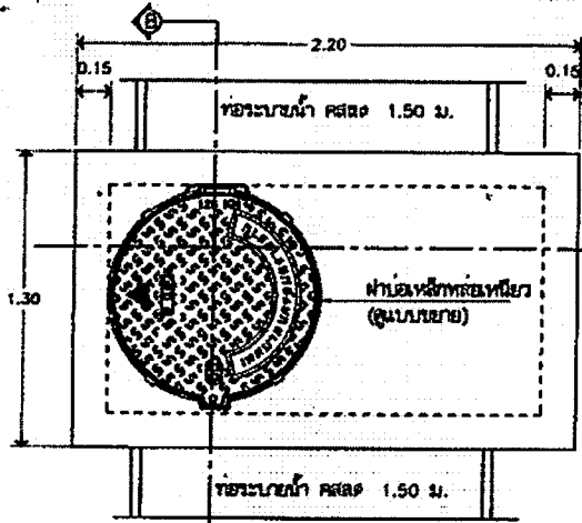
แปลนระบระบายน้ำในวิศวกรรม SCALE 1:25
