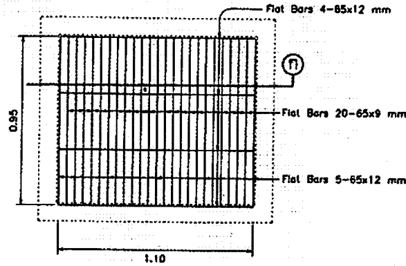
ขยาฝาท่อชัก EE 1:20
