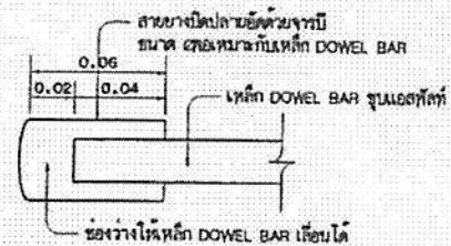
รูปตัด (1) SCALE 1:2.5
