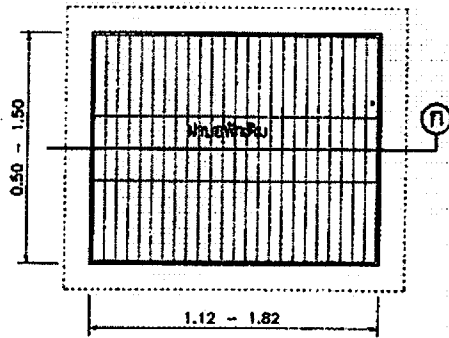
แป้นฝาท่อชัก A,B,C,D,E,F 1:20
