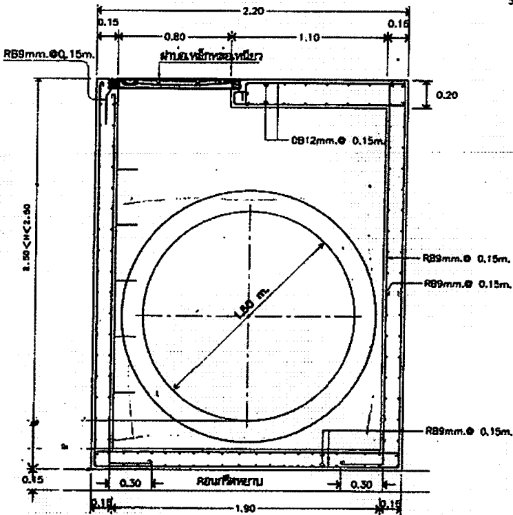
รูปตัด A SCALE 1:25
