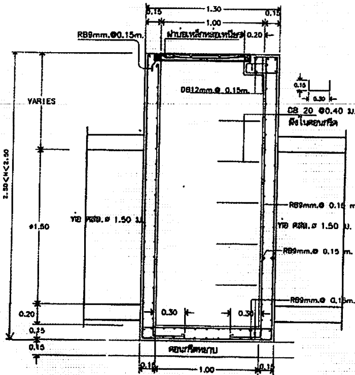
รูปตัด B SCALE 1:25
