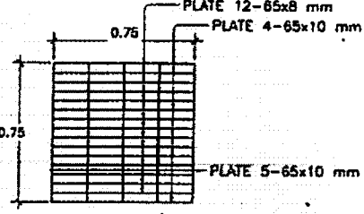
แบบขยายฝากรอบน้ำ SCALE 1:25
