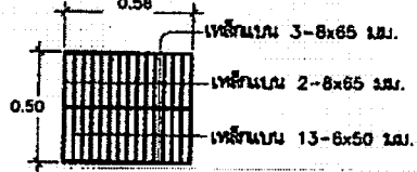
แบบขยายฝากรอบน้ำ SCALE 1:25
