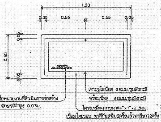
ค้ำหลังป้ายโครงการ SCALE 1:20
