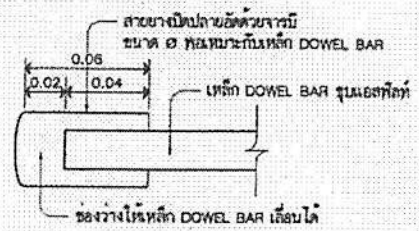
รูปตัด SCALE 1:25
