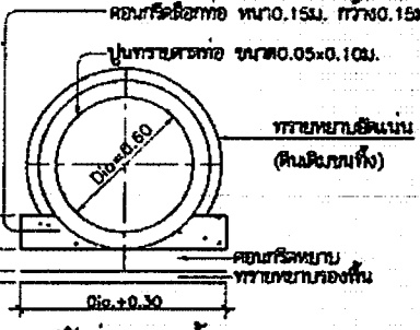
รูปตัดของระบายน้ำ SCALE 1:25
