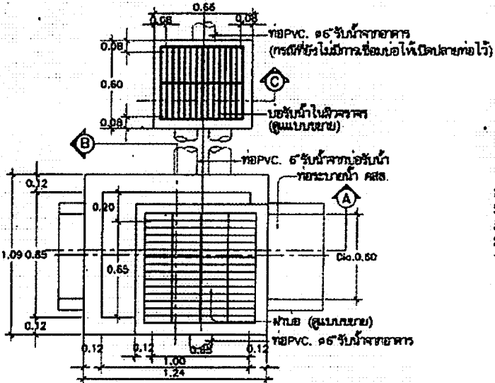
แบบระบระบายน้ำในผิวจราจร SCALE 1:25
