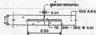
LONGITUDINAL JOINT 1:20
