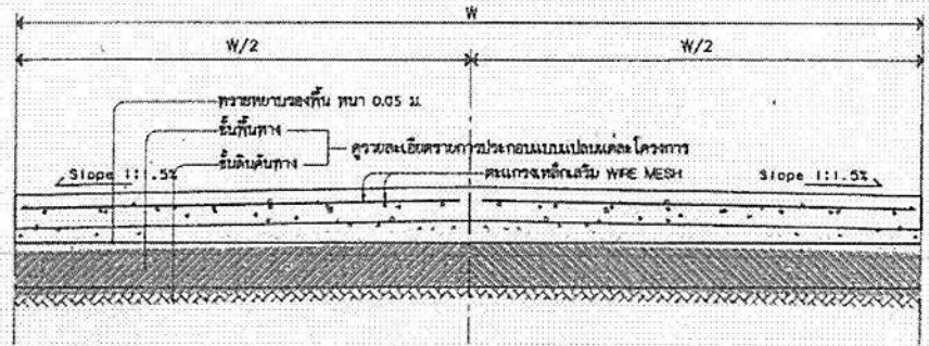
รูปตัด SCALE 1:25
