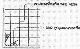
ขยายการเสริมเหล็กคานวาง SCALE 1:50
