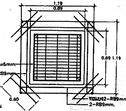
แบบขยายเหล็กเสริมรอบฝากรอบน้ำ SCALE 1:25
