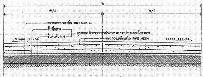
รูปตัด SCALE 1:25
