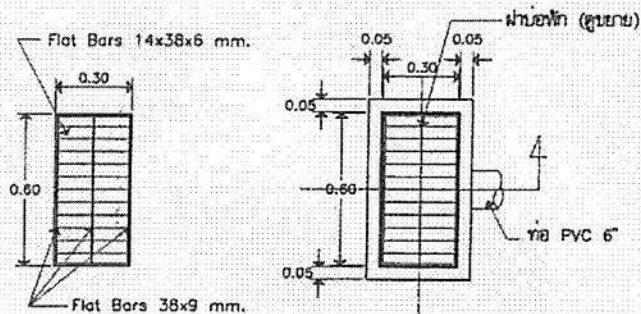
ขยายฝาท่อชักน้ำ H SCALE 1:20
