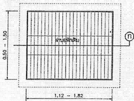
แปลนบ่อพัก A,B,C,D,E,F 1:20
