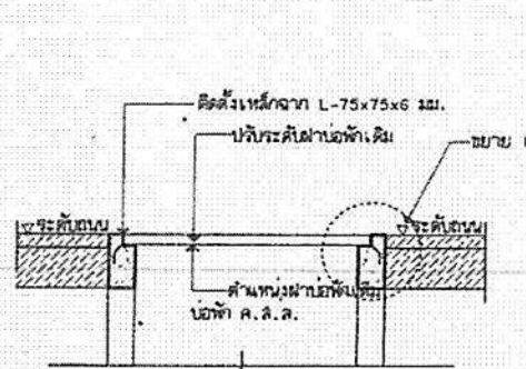
รูปตัด ก มาตราส่วน 1:25
