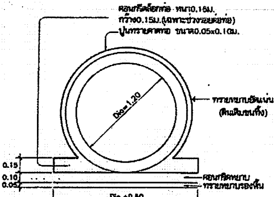
รูปตัดของระบระบายน้ำ SCALE 1:25
