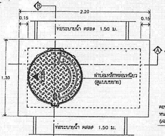
แปลนระบระบายน้ำในวงจรร
