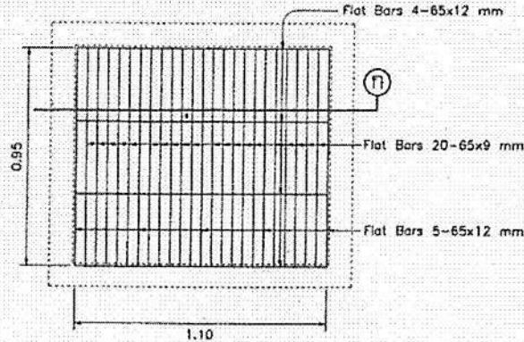
ขยายฝาท่อชัก EE 1:20
