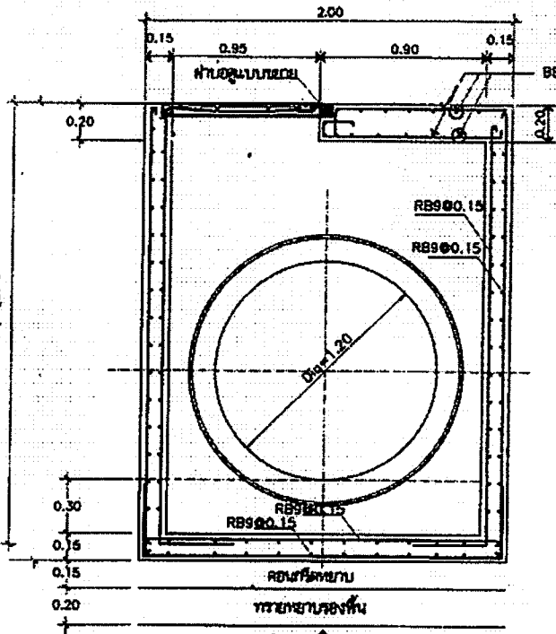
รูปตัด B-B SCALE 1:25
