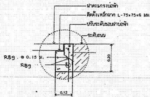
ขยาย 1 มาตราส่วน 1:20
