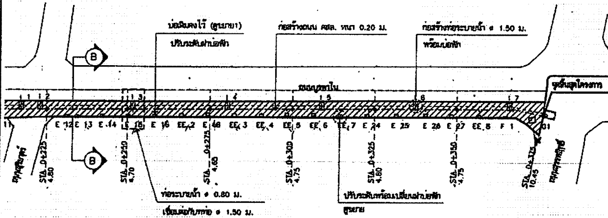
แปลนก่อสร้างถนน ค.ส.ส. และระบบระบายน้ำ
