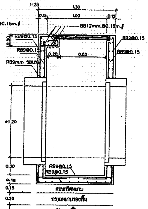
รูปตัด A-A SCALE 1:25
