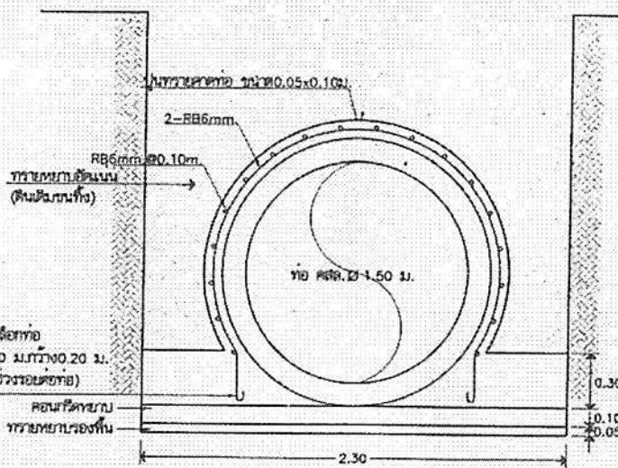
รูปตัดที่เอระบายน้ำ
