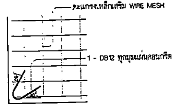
ขยายการเสริมเหล็กคานยาว SCALE 1:50
