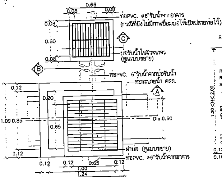
แปลนระบบระบายน้ำในผิวจราจร SCALE 1:25
