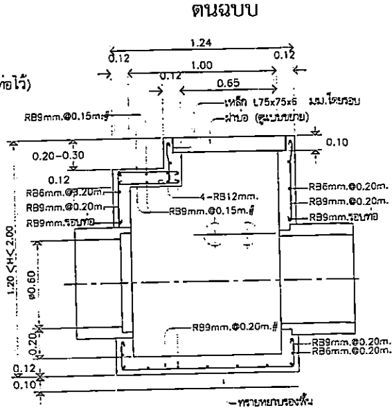
รูปตัด A SCALE 1:25
