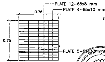
แบบขยายฝาท่อ SCALE 1:25
