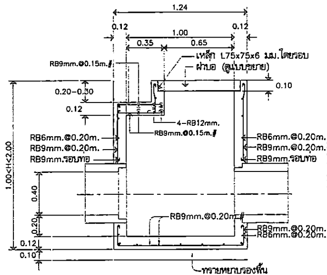
รูปตัด A-A SCALE 1:25
