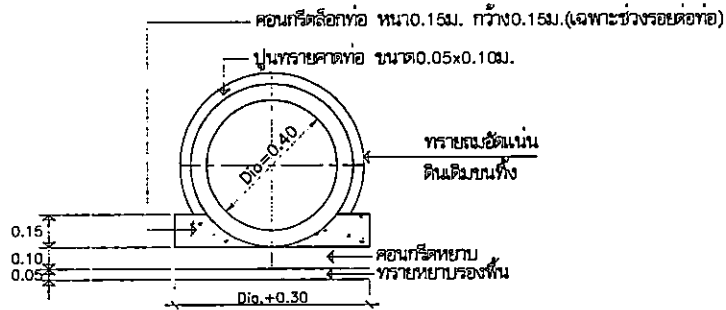
รูปตัดท่อระบายน้ำ SCALE 1:25
