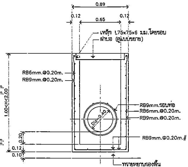
รูปตัด B-B SCALE 1:25
