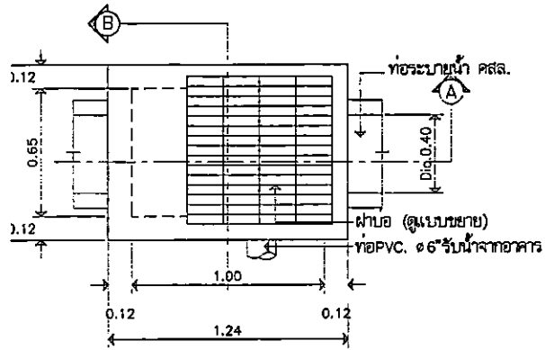
แปลนระบบระบายน้ำในผิวจราจร SCALE 1:25
