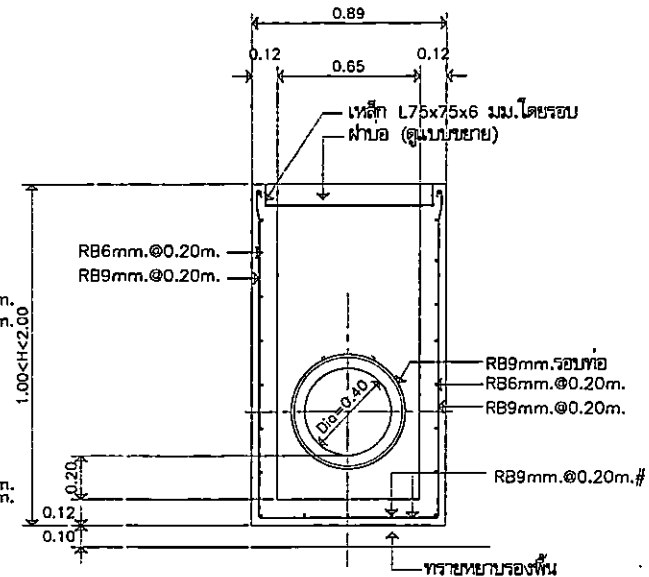
รูปตัด B SCALE 1:25
