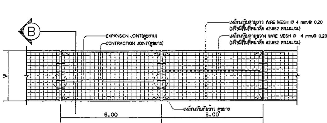
แปลนถนน ค.ส.ล. (หนา 0.15 ม.) SCALE 1:100
